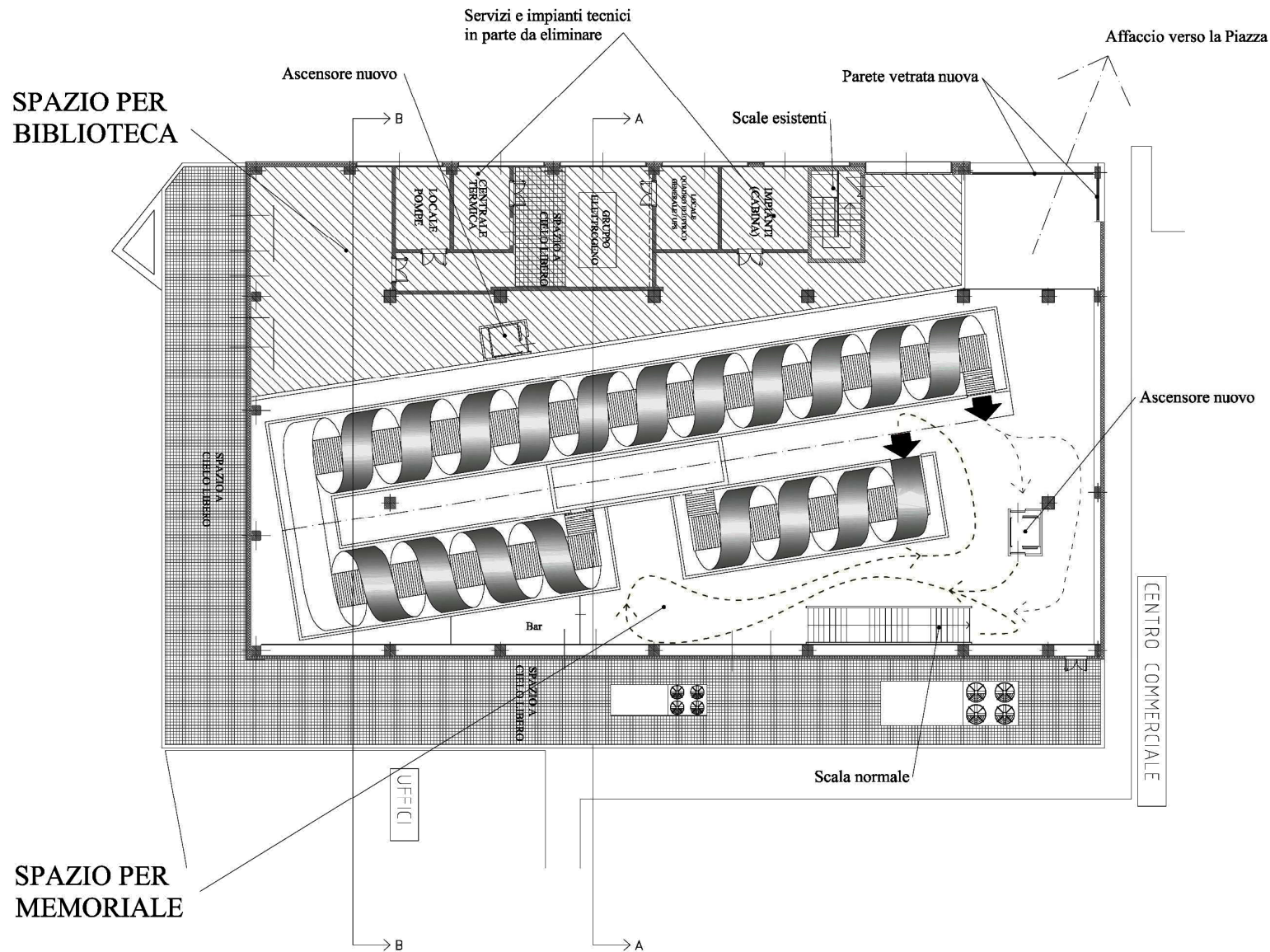
Memorial nell'edificio EX3 1:200
